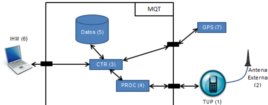
Figura 1. Esquema de conexión y equipo para evaluar la calidad del servicio de telefonía móvil 2 mediante drive test .
