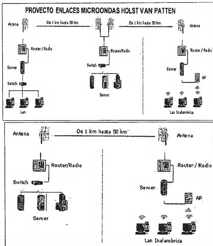
Figura 1. Topología de Red para conexiones punto a multipunto y punto a punto.
