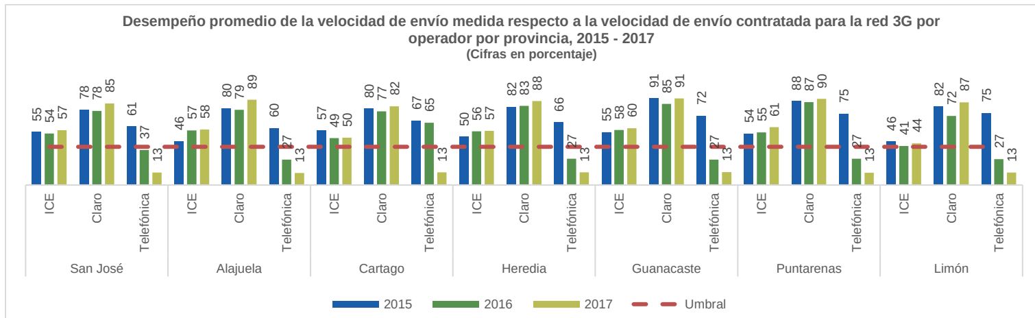
Gráfico 32 Desempeño promedio de la velocidad de envío medida respecto del umbral (40%) para la red 3G por operador por provincia, para los años 2015, 2016 y 2017
