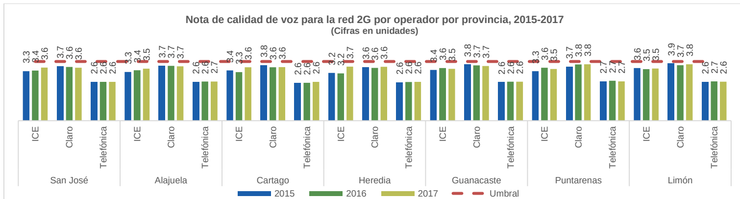
Gráfico 21 Nota de calidad de voz respecto del umbral (4 MOS 27 ) para la red 2G por operador por provincia, para los años 2015, 2016 y 2017
