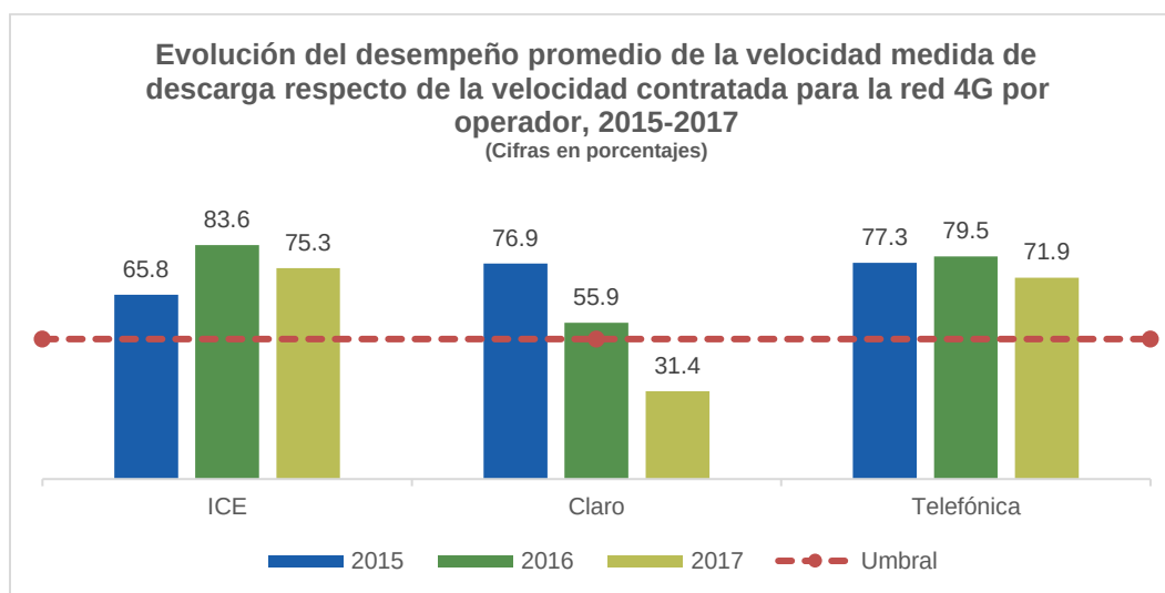
Gráfico 12 Evolución del desempeño promedio de la velocidad medida de descarga respecto del umbral (50%) para la red 4G por operador, para los años 2015, 2016 y 2017
