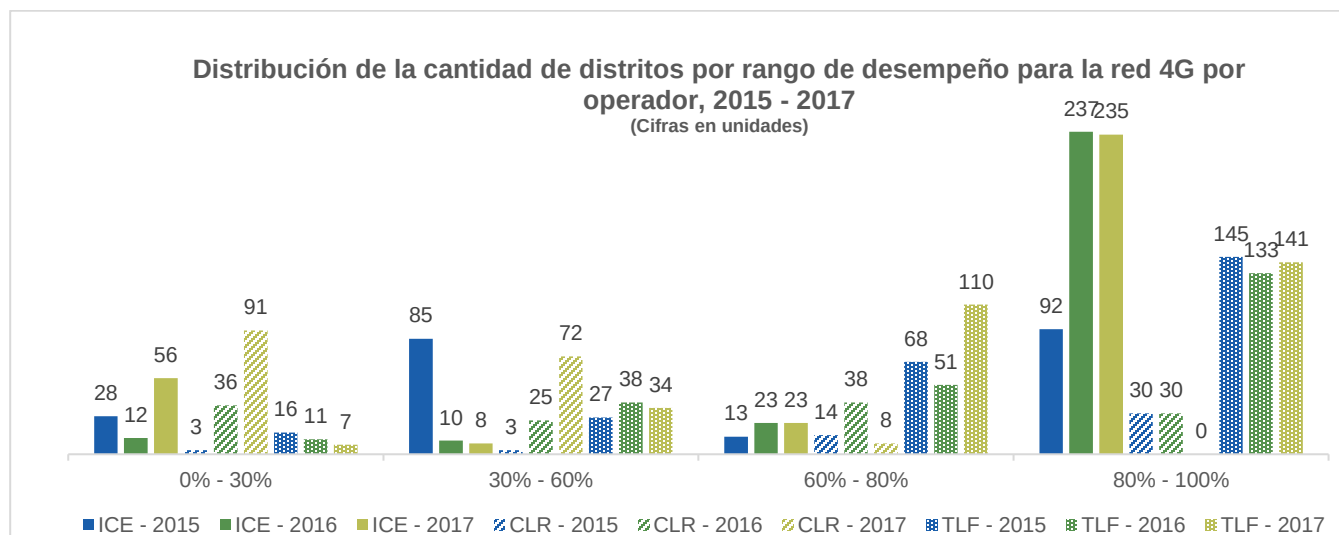
Gráfico 13 Distribución de la cantidad de distritos por rango de desempeño para la red 4G por operador, para los años 2015, 2016 y 2017
