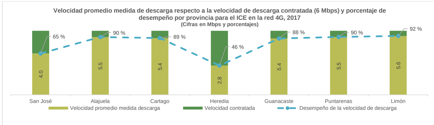
Gráfico 29 Velocidad promedio medida de descarga respecto de la velocidad de descarga contratada (6Mbps) y el porcentaje de desempeño para la red 4G del operador ICE por provincia, año 2017
