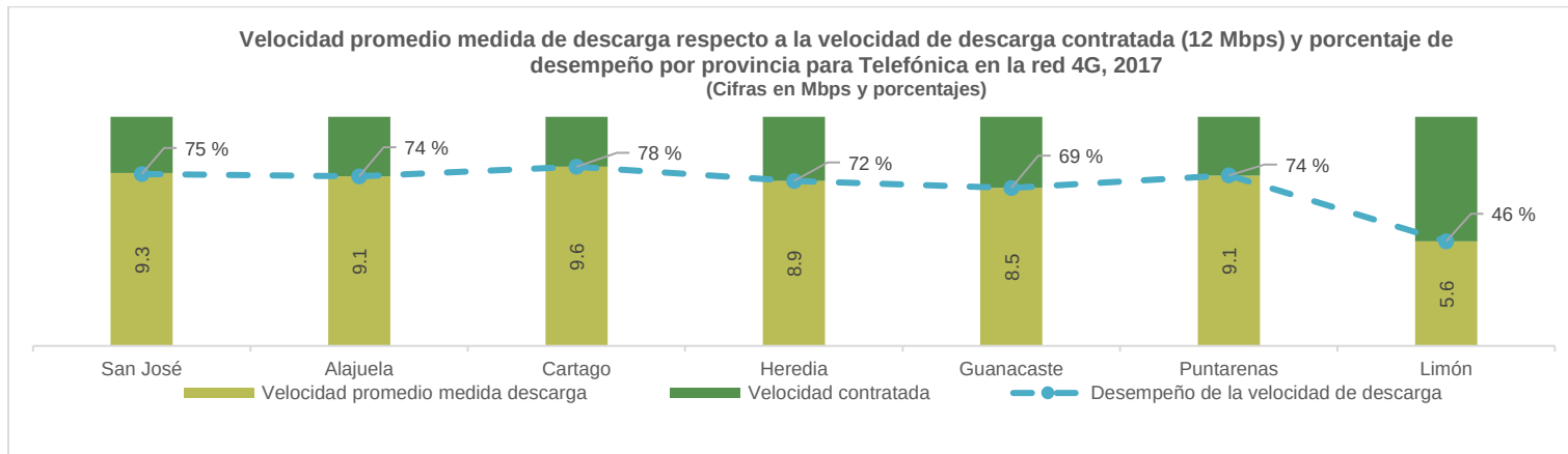
Gráfico 30 Velocidad promedio medida de descarga respecto de la velocidad de descarga contratada (12Mbps) y el porcentaje de desempeño para la red 4G del operador TLF por provincia, año 2017
