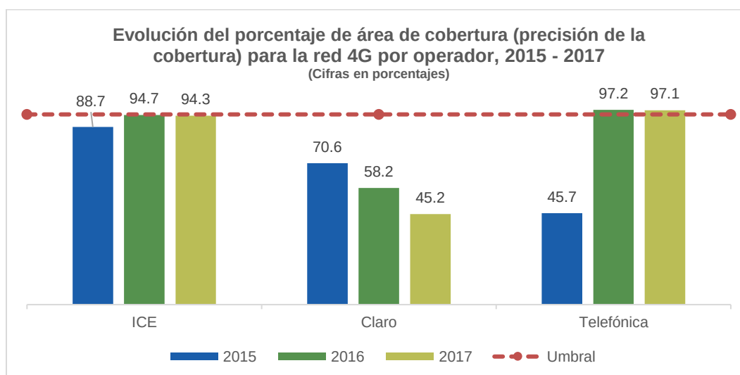
Gráfico 5 Evolución del porcentaje de área de cobertura (precisión de la cobertura) respecto del umbral (95%) para la red 4G por operador, para los años 2015, 2016 y 2017
