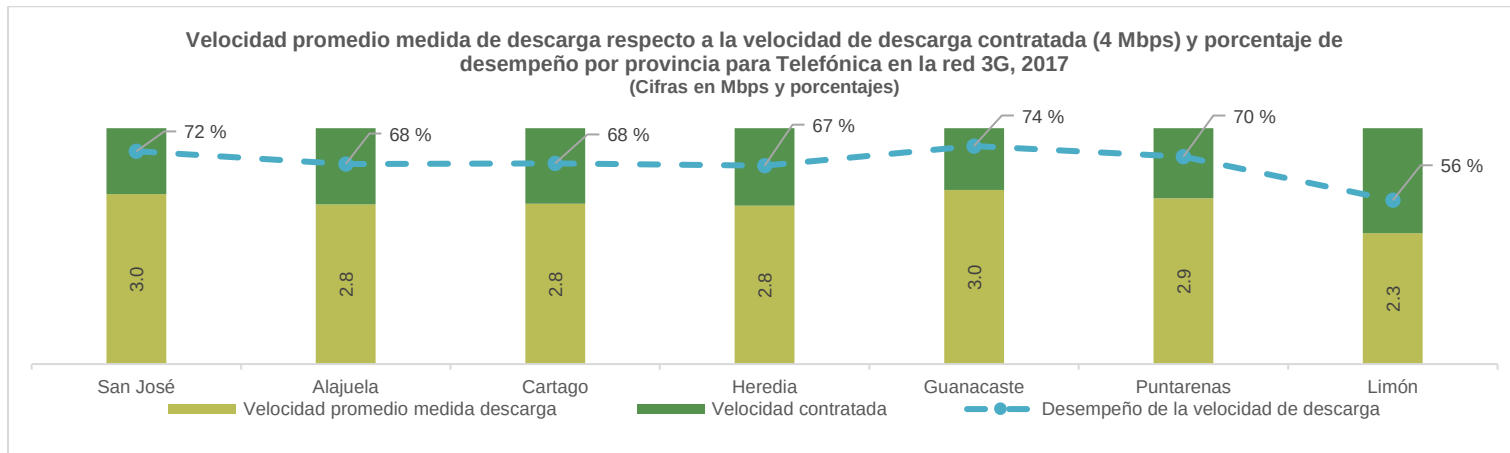
Gráfico 26 Velocidad promedio medida de descarga respecto de la velocidad de descarga contratada (4Mbps) y el porcentaje de desempeño para la red 3G del operador TLF por provincia, año 2017
