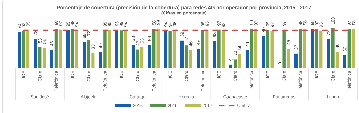
Gráfico 18 Porcentaje de cobertura (precisión de la cobertura) respecto del umbral (95%) para la red 4G por operador por provincia, para los años 2015, 2016 y 2017
