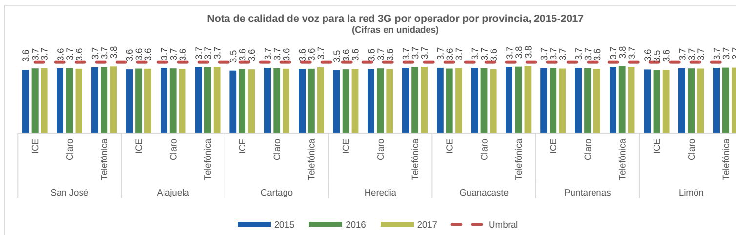
Gráfico 22 Nota de calidad de voz respecto del umbral (4 MOS 28 ) para la red 3G por operador por provincia, para los años 2015, 2016 y 2017
