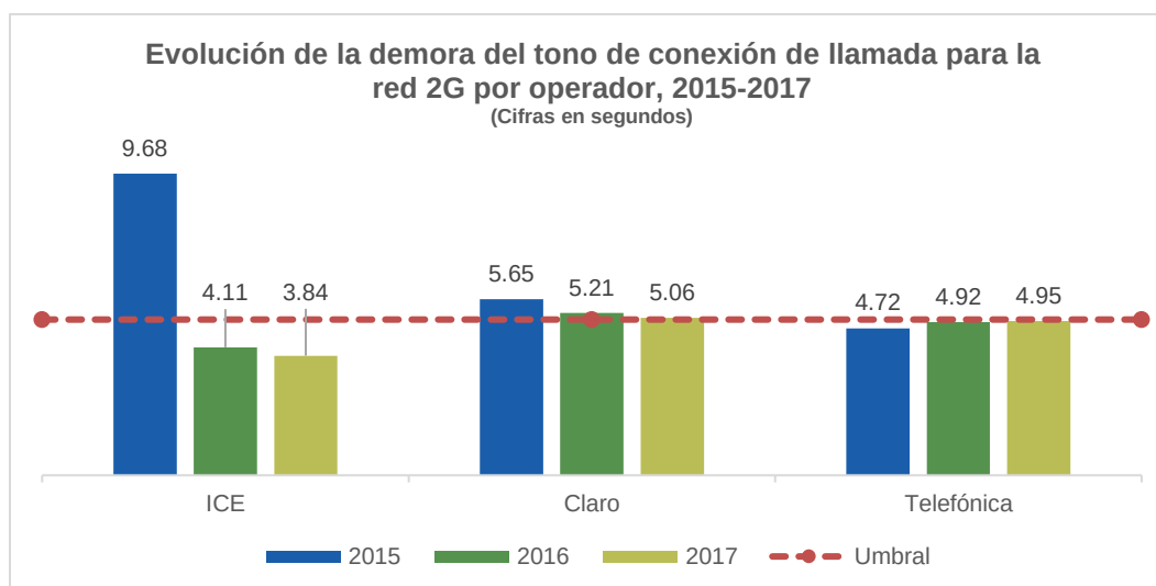
Gráfico 6 Evolución de la demora del tono de conexión de llamada respecto del umbral (5 segundos) para la red 2G por operador, para los años 2015, 2016 y 2017
