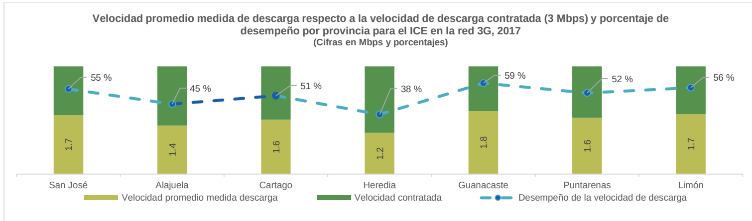
Gráfico 25 Velocidad promedio medida de descarga respecto de la velocidad de descarga contratada (3Mbps) y el porcentaje de desempeño para la red 3G del operador ICE por provincia, año 2017
