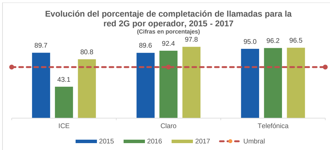
Gráfico 1 Evolución del porcentaje de completación de llamadas respecto del umbral (70%) para la red 2G por operador, para los años 2015, 2016 y 2017
