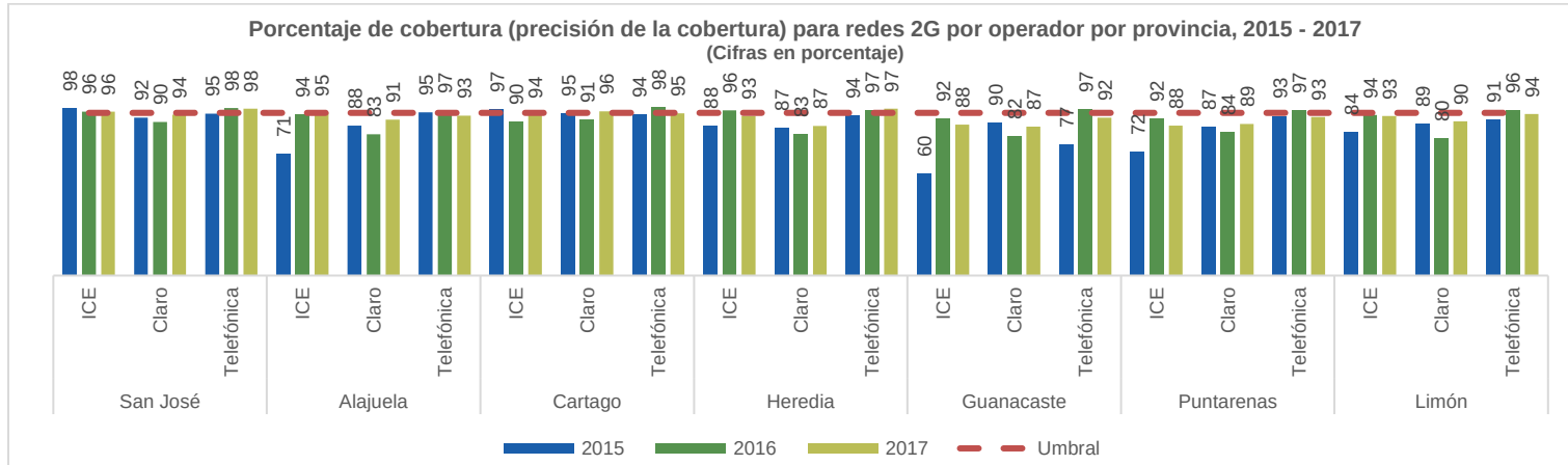
Gráfico 16 Porcentaje de cobertura (precisión de la cobertura) respecto del umbral (95%) para la red 2G por operador por provincia, para los años 2015, 2016 y 2017
