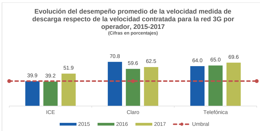
Gráfico 10 Evolución del desempeño promedio de la velocidad medida de descarga respecto del umbral (40%) para la red 3G por operador, para los años 2015, 2016 y 2017
