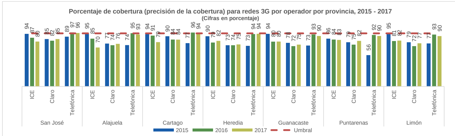
Gráfico 17 Porcentaje de cobertura (precisión de la cobertura) respecto del umbral (95%) para la red 3G por operador por provincia, para los años 2015, 2016 y 2017
