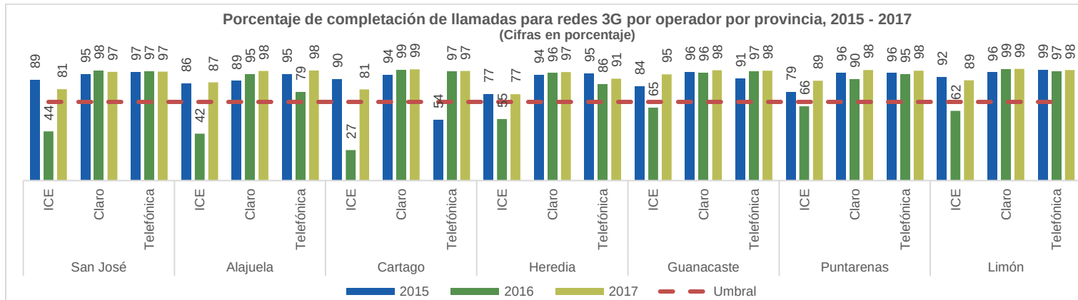
Gráfico 15 Porcentaje de completación de llamadas respecto del umbral (70%) para la red 3G por operador por provincia, para los años 2015, 2016 y 2017
