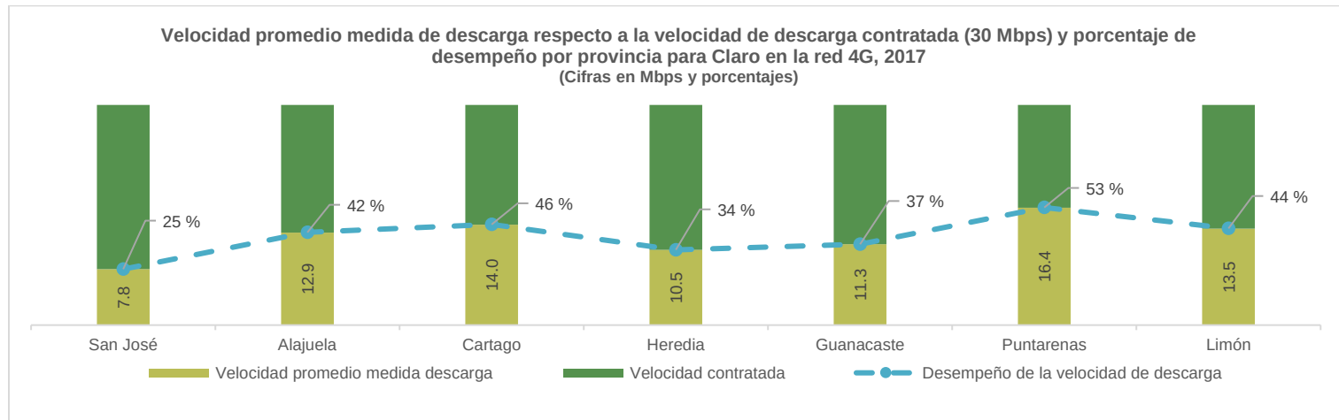
Gráfico 28 Velocidad promedio medida de descarga respecto de la velocidad de descarga contratada (30Mbps) y el porcentaje de desempeño para la red 4G del operador CLR por provincia, año 2017
