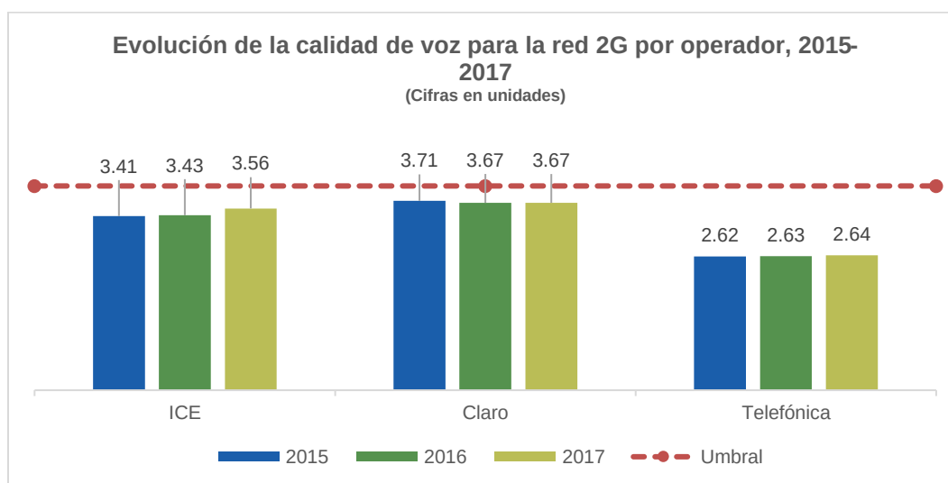
Gráfico 8 Evolución de la calidad de voz respecto del umbral (4 MOS 19 ) para la red 2G por operador, para los años 2015, 2016 y 2017
