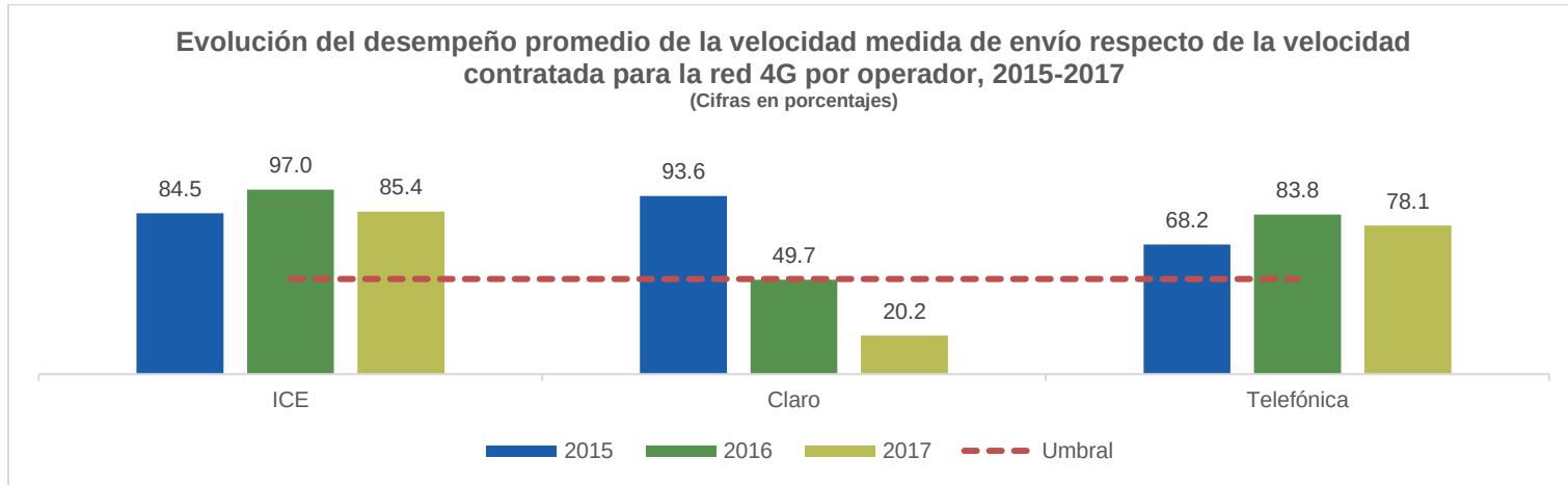
Gráfico 33 Evolución del desempeño promedio de la velocidad medida de envío respecto al umbral (50%) para la red 4G por operador, para los años 2015, 2016 y 2017
