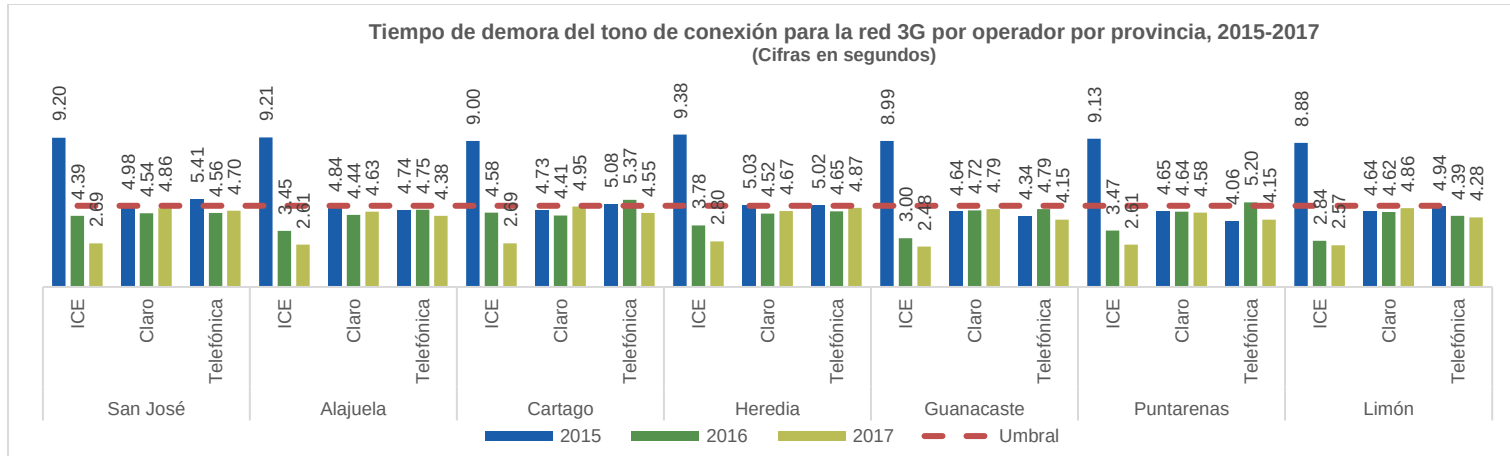
Gráfico 20 Tiempo de establecimiento de llamada respecto del umbral (5 segundos) para la red 3G por operador por provincia, para los años 2015, 2016 y 2017
