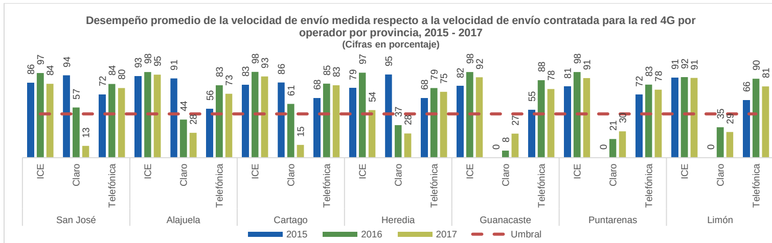
Gráfico 34 Desempeño promedio de la velocidad de envío medida respecto del umbral (50%) para la red 4G por operador por provincia, para los años 2015, 2016 y 2017
