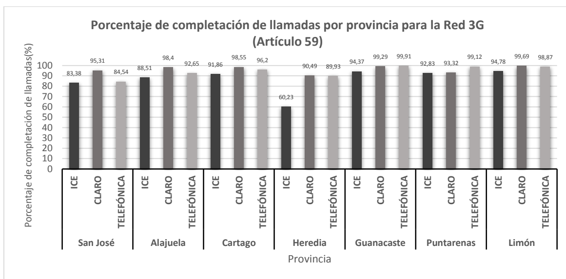
Figura 4. Resultados de porcentaje de completación de llamadas por provincia para la red 3G de los operadores ICE, CLR y TLF.
