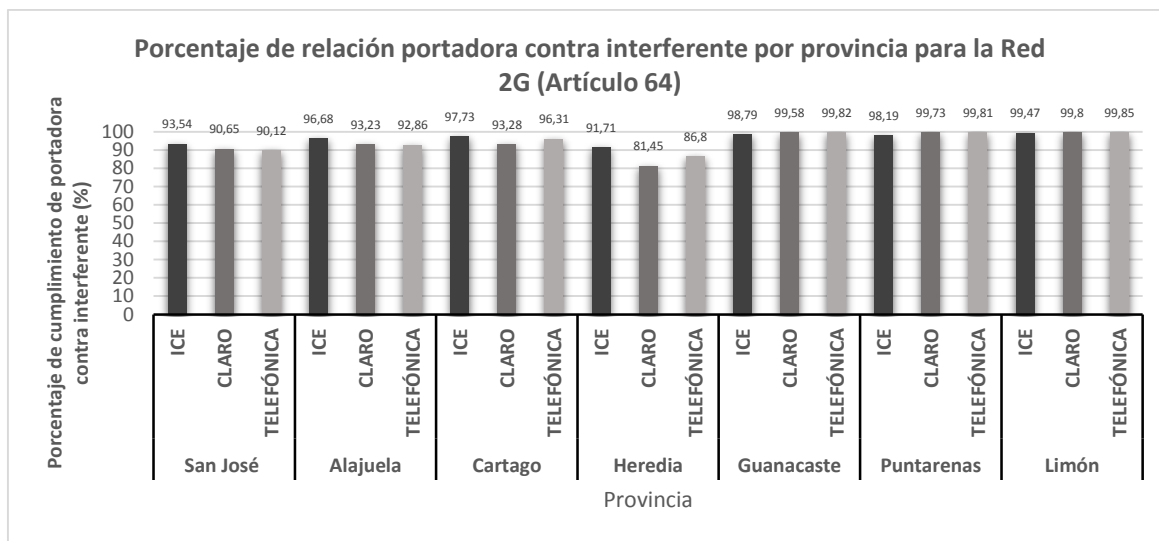
Figura 7. Resultados de portadora contra interferente detallado por provincia para la Red 2G del ICE, CLR y TLF.
