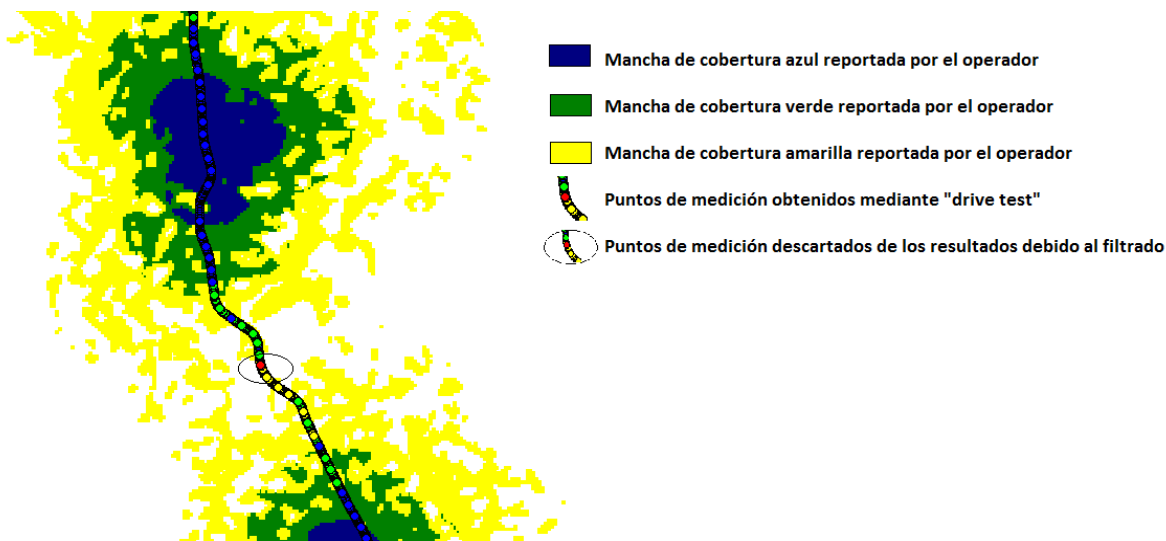
Figura 2. Ilustración del proceso de filtrado de los datos de drive test obtenidos y las manchas de cobertura reportadas por el operador.
