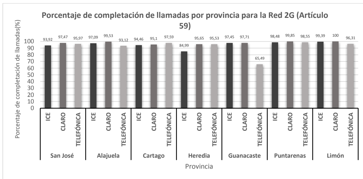
Figura 3. Resultados de porcentaje de completación de llamadas por provincia para la red 2G de los operadores ICE, CLR y TLF.
