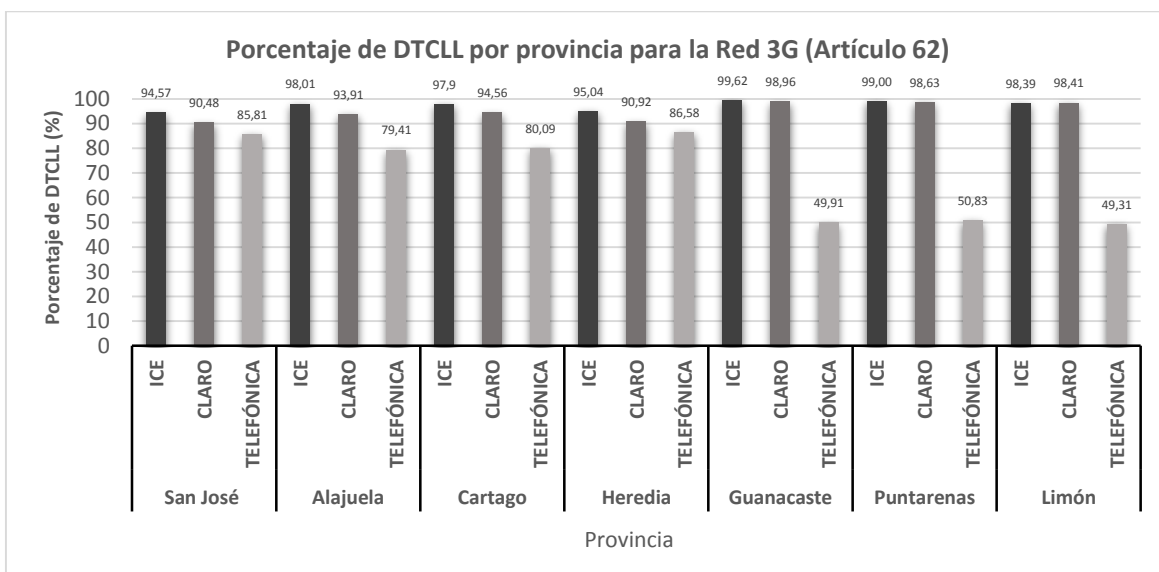
Figura 10. Resultados de DTCLL detallado por provincia para la Red 3G del ICE, CLR y TLF.
