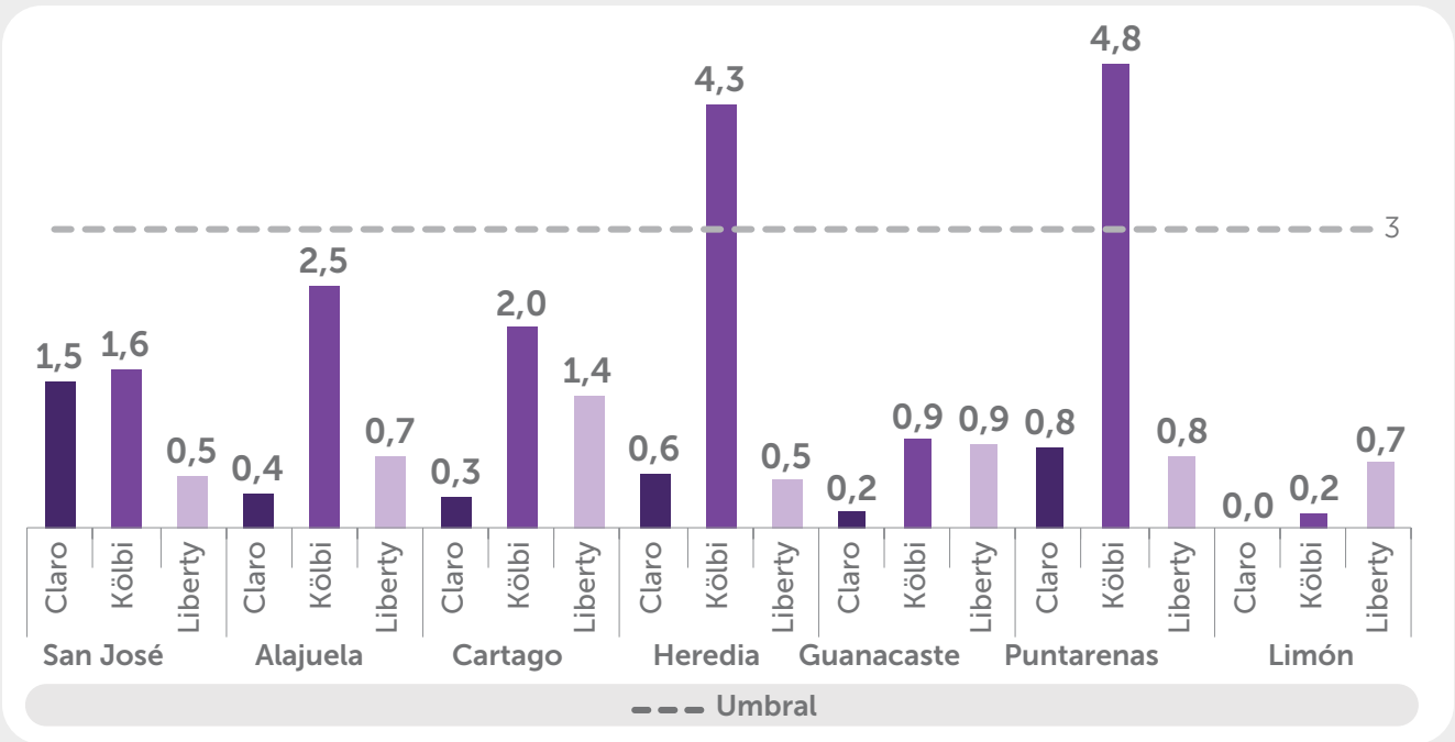
GRÁFICO 3. Porcentaje de llamadas no exitosas en la red 3G por provincia, para el año 2025 (Cifras en porcentajes)
