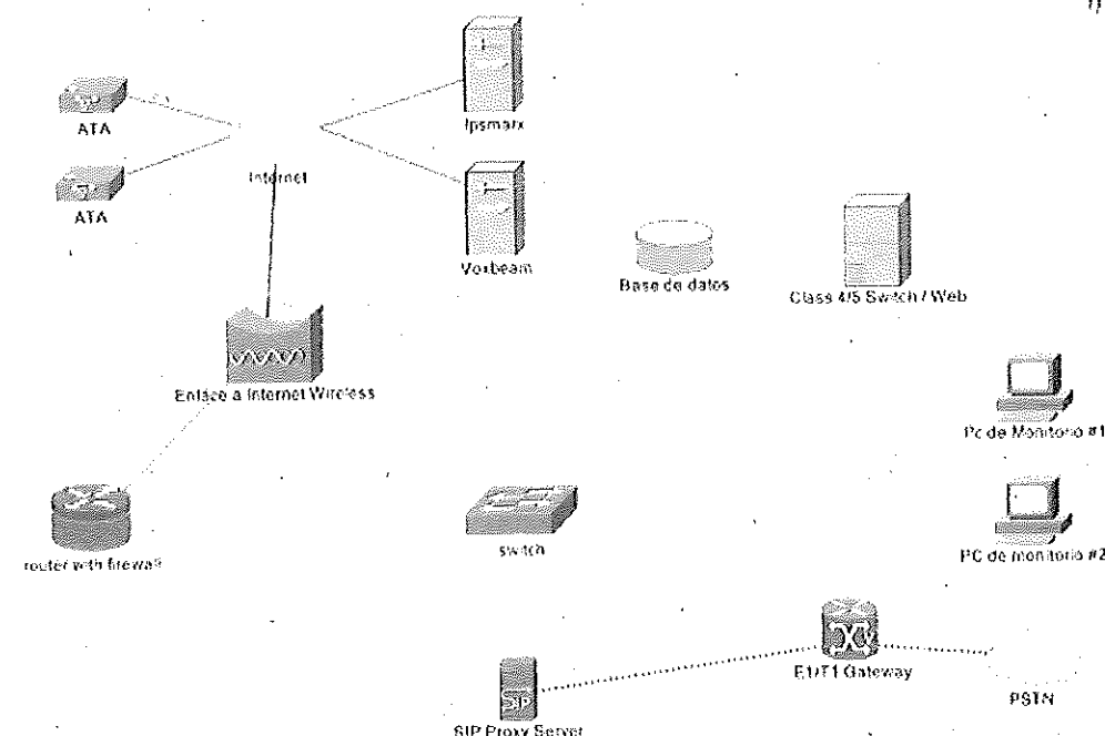
Figura 2. Diagrama de red Comunicaciones Integrales ANI, S.A.
