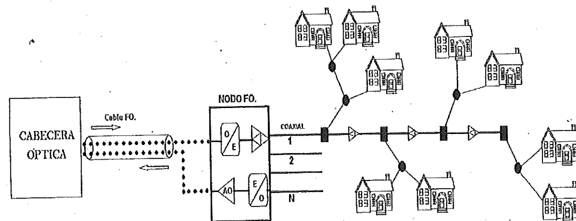
Figura 1. Topología de red para el servicio de Televisión por Suscripción por medio de red HFC
