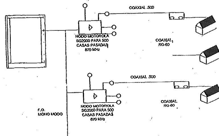
Figura 3. Diagrama de red para servicio de Televisión por Suscripción proporcionado por medio de una red de tipo HFC
