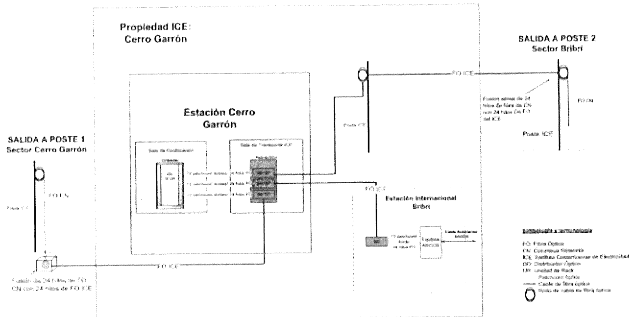
Figura 3. Diagrama técnico de conexión para acceso por parte de C&W.
