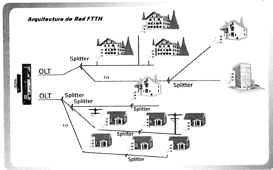
Figura 1. Diagrama de la Arquitectura de red. Aportado por Cable Suisa S.A.
