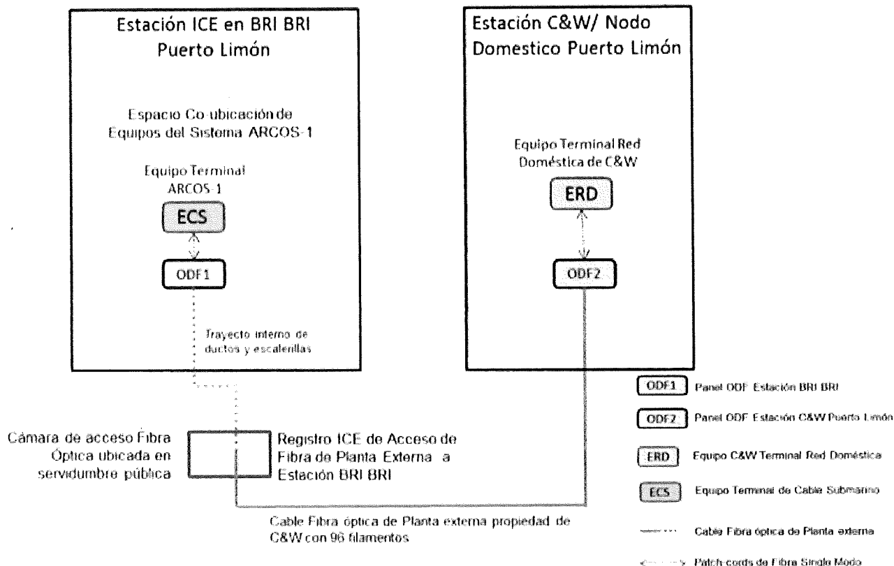
Figura 1. Diagrama técnico aportado por C&W en relación con la solicitud realizada al ICE para acceder a la estación BRI BRI. (visible a folio 32 del expediente administrativo).
