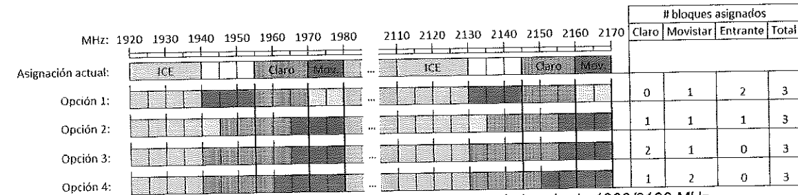
Figura 2. Opciones de reordenamiento de espectro en la banda de 1900/2100 MHz
