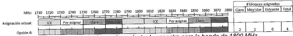
Figura 3. Propuesta de reordenamiento de espectro para la banda de 1800 MHz
