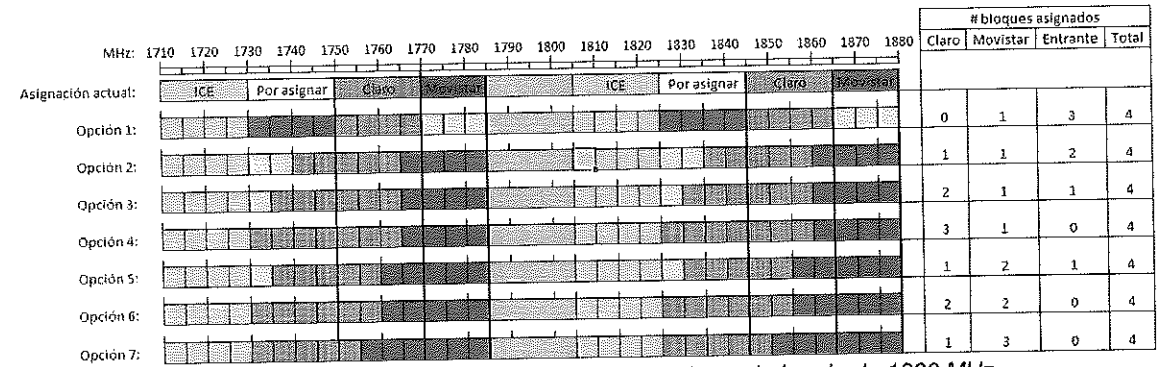
Figura 1. Opciones de reordenamiento de espectro en la banda de 1800 MHz
