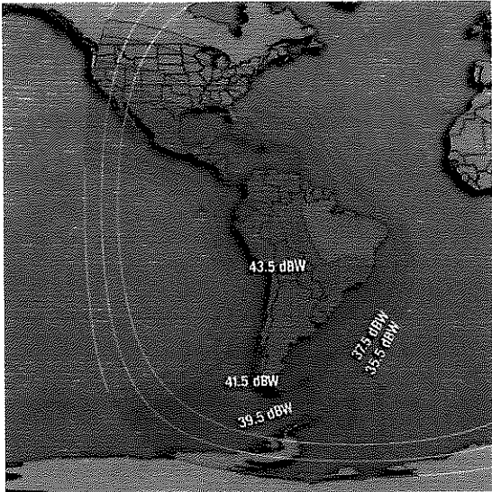
Figura 1. Área de cobertura para el satélite Intelsat 14 en la banda C. 1
