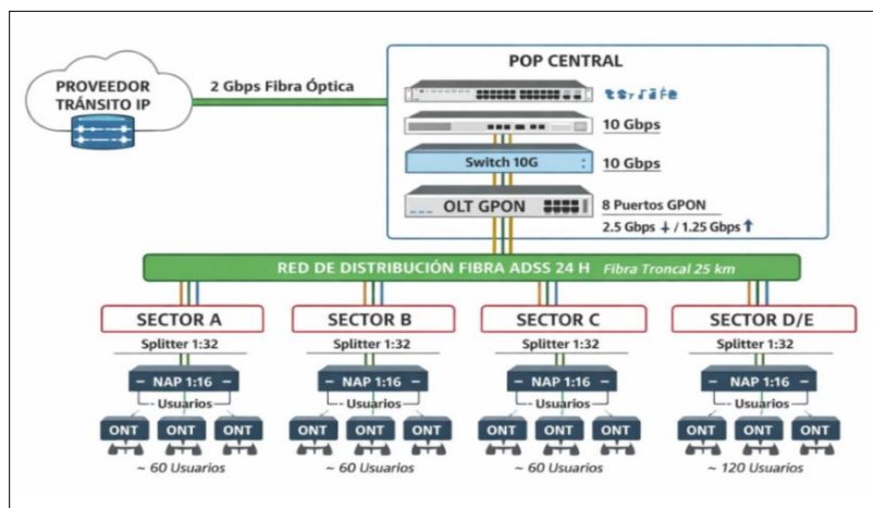
Figura 4. Diagrama de red aportado por el señor GILBERT DÍAZ PARRA .
